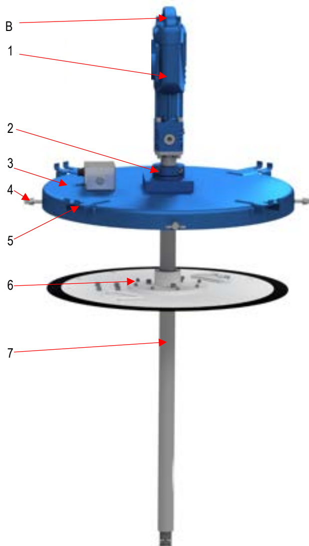
Bild 14 (Darstellung ohne Motor)
